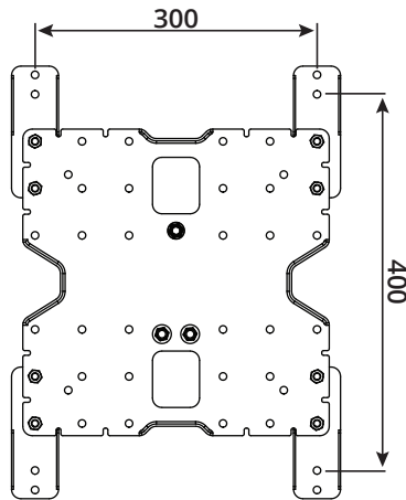
VESA: 300X400
