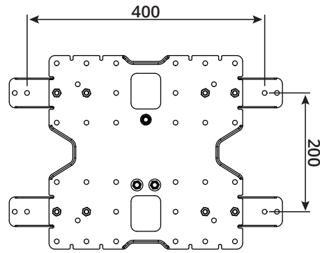
VESA: 400X200
