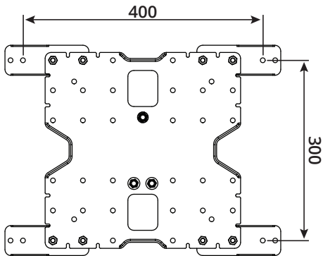
VESA: 400X300
