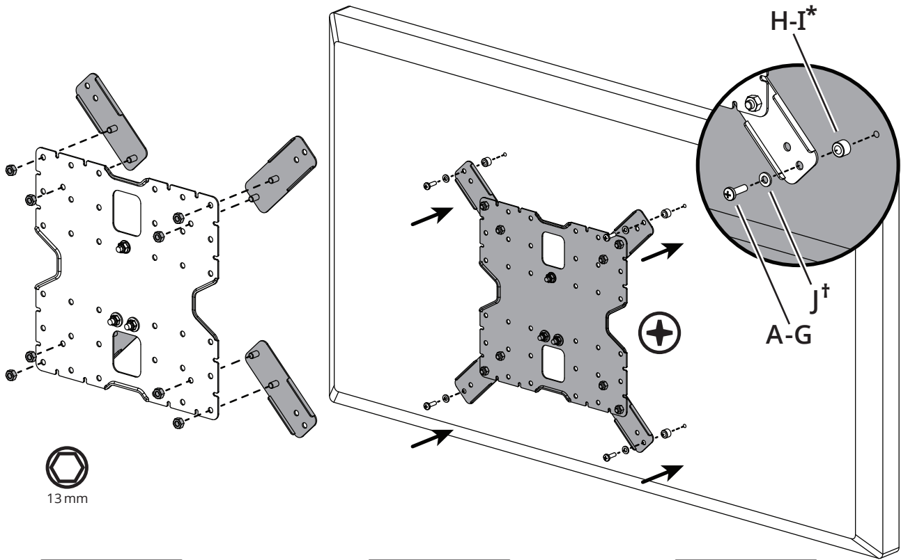
VESA: 400X400
